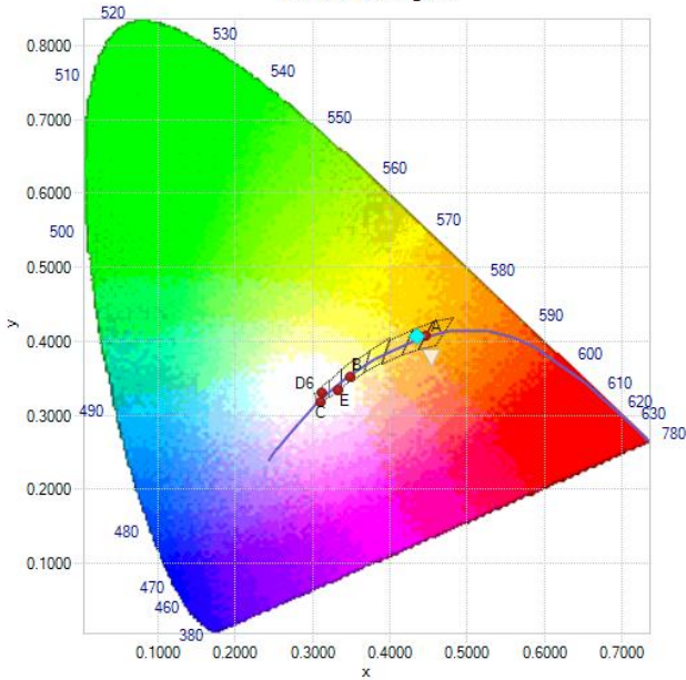
CIE 1931, 2 Degree
